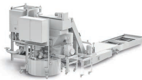
Convoyeur avec broyeur de copeaux, station de repompage RKR et dispositif haute pression DHS
