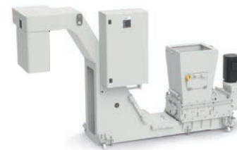
Convoyeur avec broyeur de copeaux
