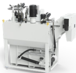
Filtro a tamburo in depressione VRF
