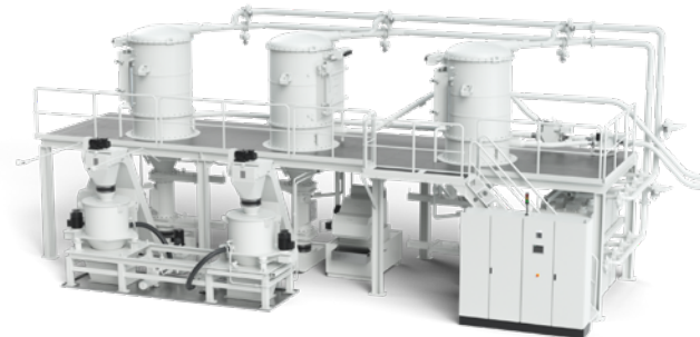
Sistema a tecnica di aspirazione
