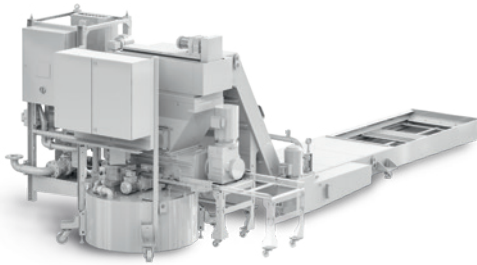
Convogliatore con trituratore trucioli, stazione di rilancio RKR e stazione di overboost DHS
