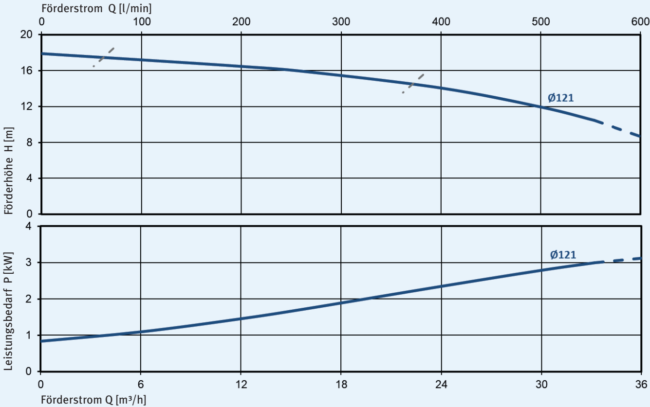
Kennlinien für 2.900 min -1 , 50 Hz, 1 mm 2 /s
