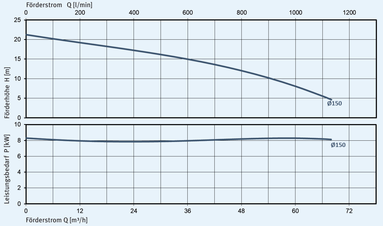
Kennlinien für 3.500 min -1 , 60 Hz, 1 mm 2 /s
