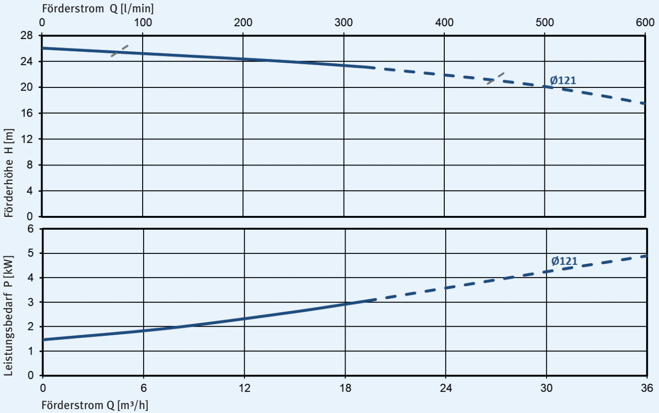
Kennlinien für 3.500 min -1 , 60 Hz, 1 mm 2 /s
